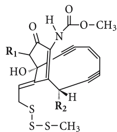
Esperamicin A_1
