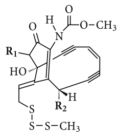
Calicheamicin \gamma_1
