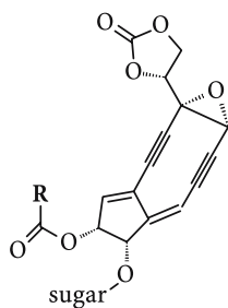
Neocarzinostatin
