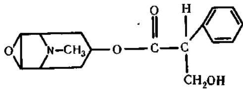
Скополамин
