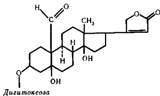
Эризимин
