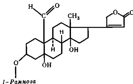
Конваллятоксин
