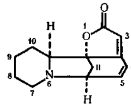
Секуринин
