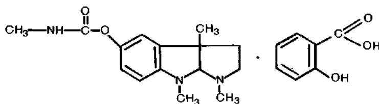
Физиостигмин
