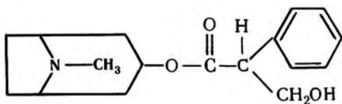
Атропин
