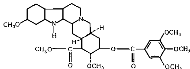
Резерпин
