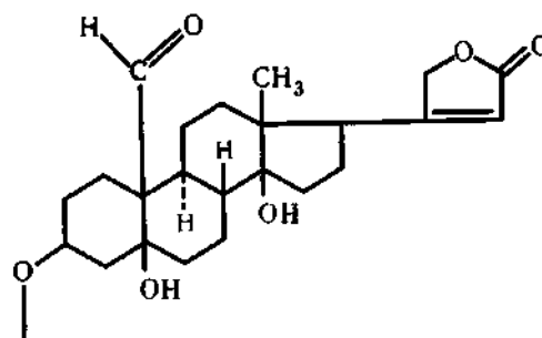
Цимароза + глюкоза
