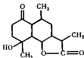
Тауремизин
