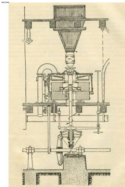
Горизонтальный жерновой постав (мельница) начала XX века. При диаметре жерновов 1245 мм и 140 об/мин производительность 285 кг муки в час. Потребляемая мощность - 6-7 л. сил (4,5-5,0 кВт).
