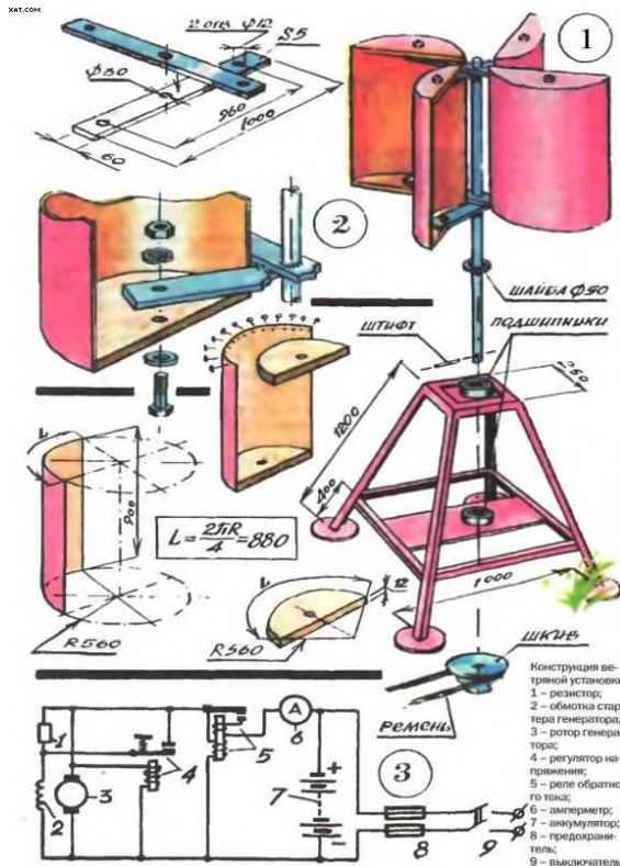
Конструкция простейшего вертикального ветряка мощностью 1 кВт 1. Внешний вид вертикального ветряка "чашечного" типа в собранном виде 2. Габаритные размеры важнейших элементов конструкции ветряка 3. Электрическая схема ветряка на основе 12 В автомобильного генератора
