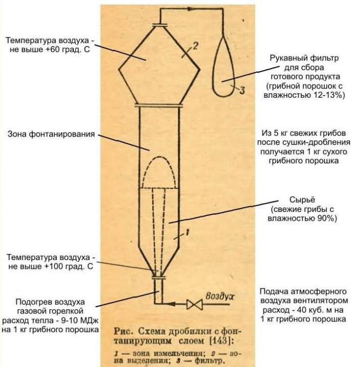
Прямоточная воздушная сушилка-дробилка для производства грибного порошка времен Второй Мировой войны. Производительность 300 кг свежих грибов в час. Мощность горелки нагревателя 170 кВт. Скорость подачи воздуха - 2400 куб. м/час.
